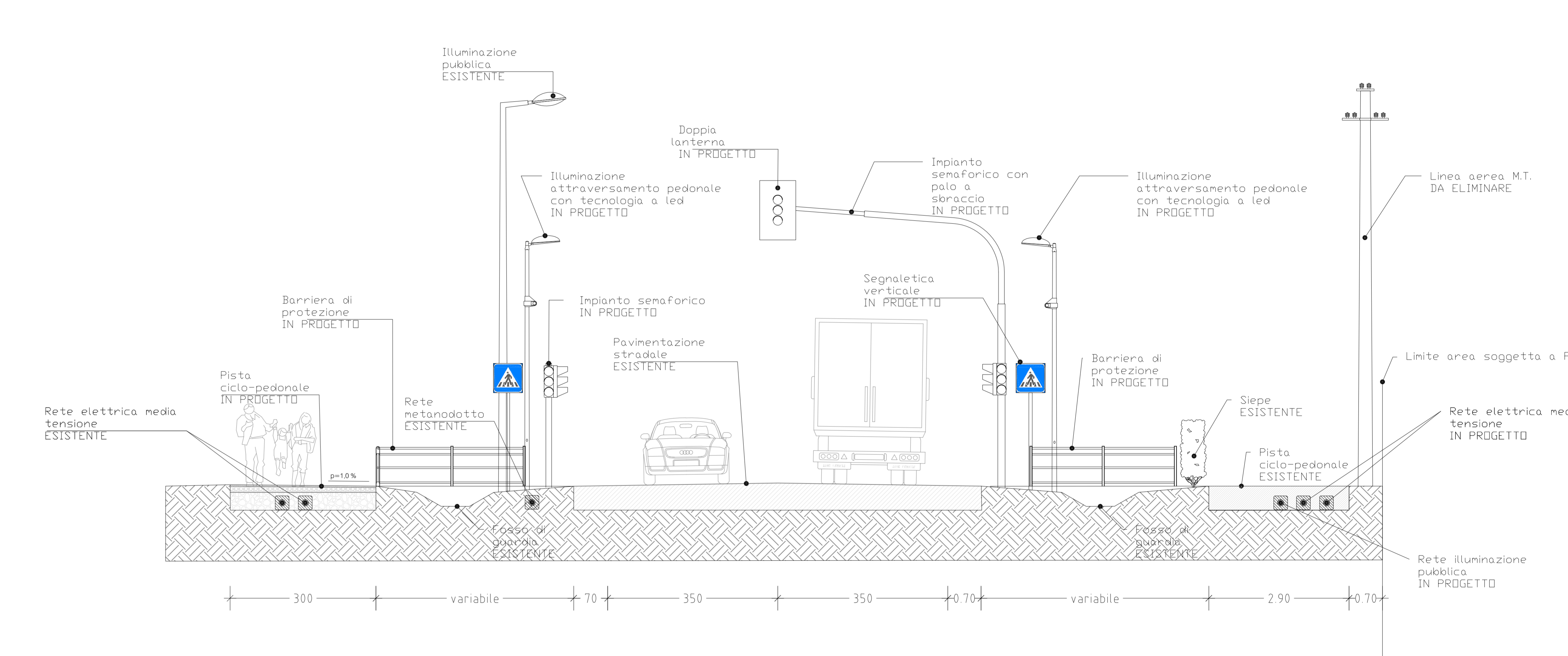
Sezione "E-E" - attraversamento pista ciclopedonale_1:50
