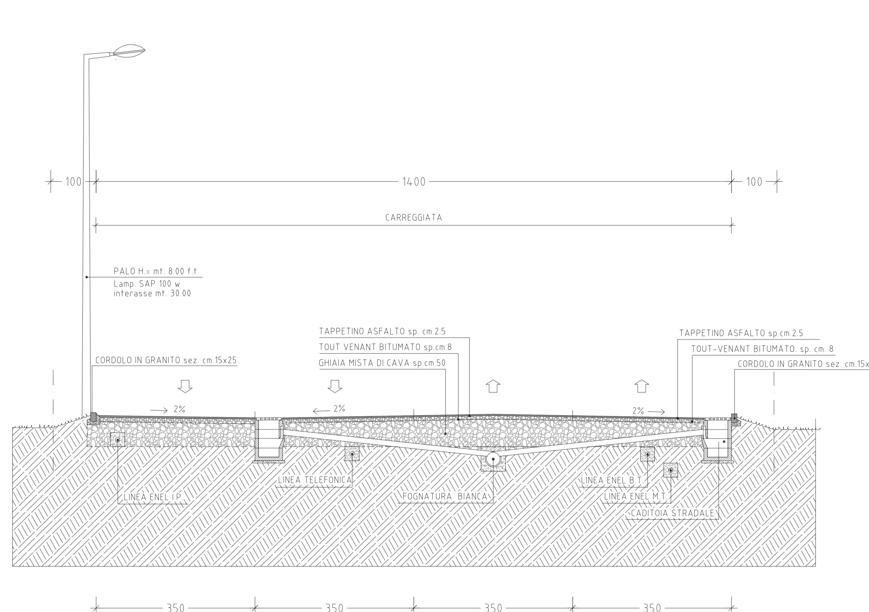
Sezione "D-D" - nuova rotatoria interna_1:50
