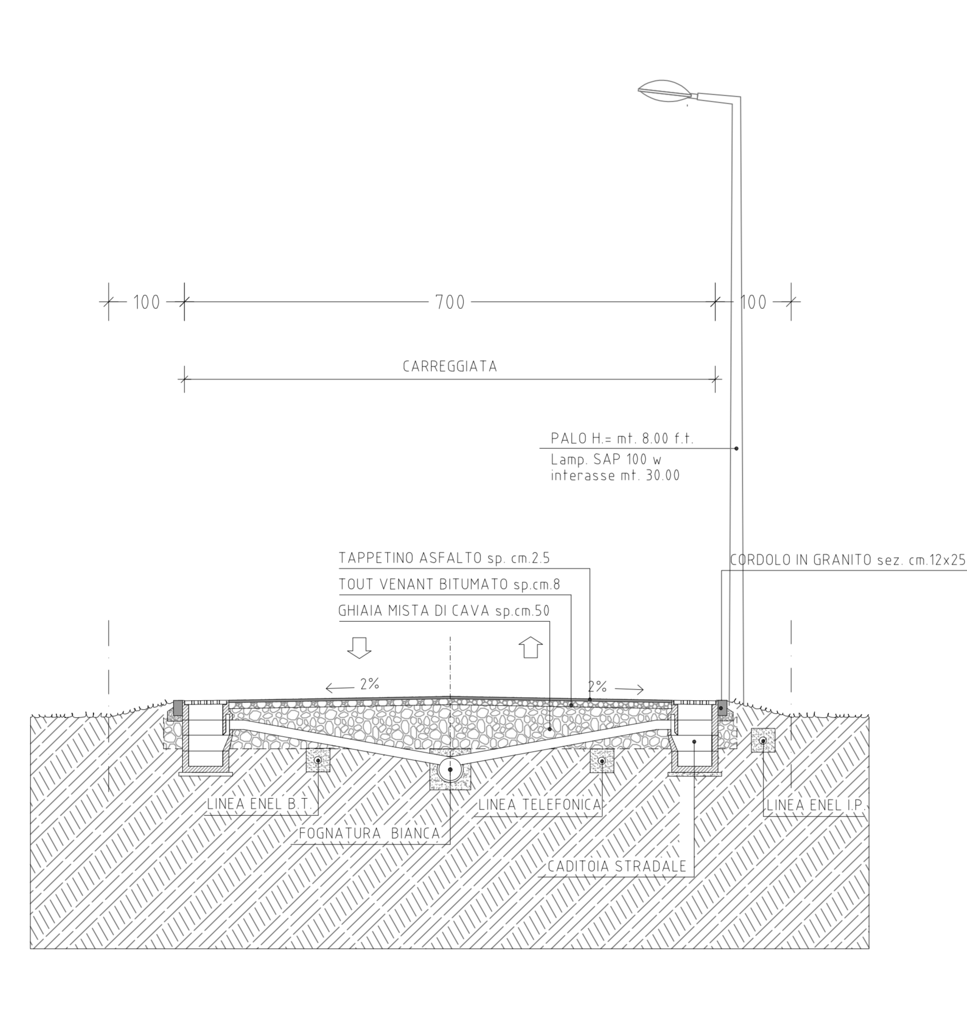
Sezione "C-C" - nuova strada di penetrazione_1:50
