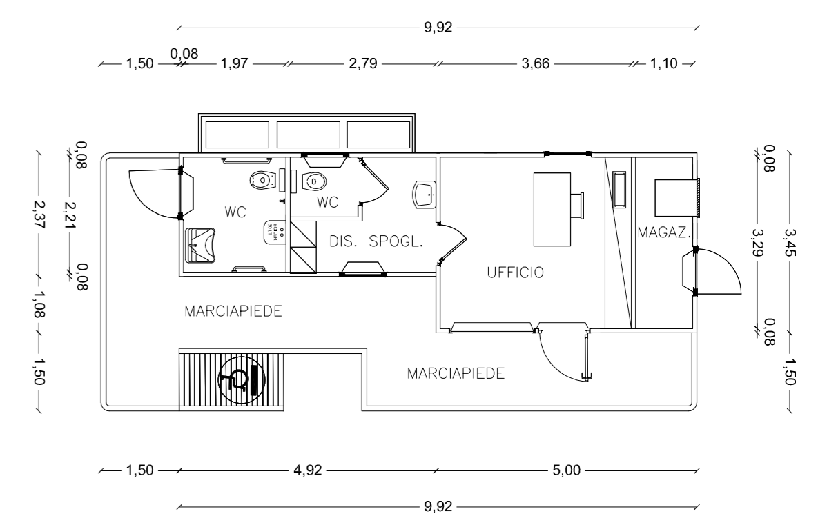
PIANTA LOCALE GESTORE scala 1:100
