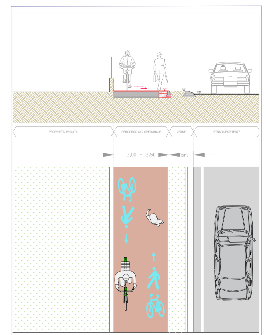
ST9 Sezione tipologica con allargamento su campo scala 1:100
