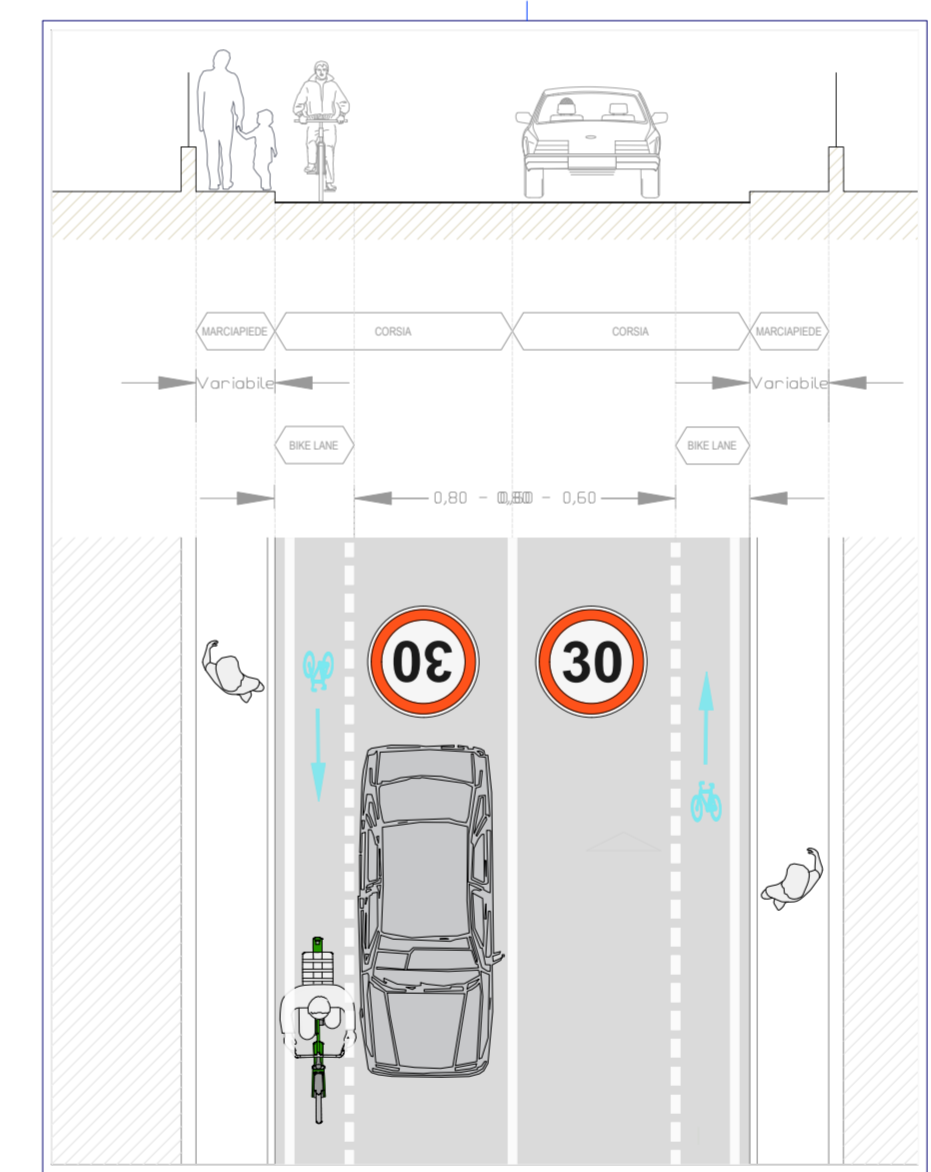
ST7 Sezione tipologica con marciapiede in quota doppio scala 1:100
