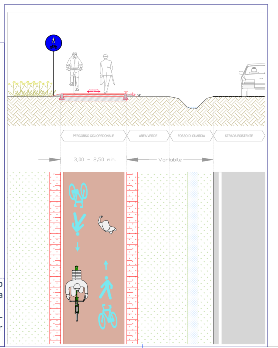
ST8 Sezione tipologica con allargamento su campo scala 1:100
